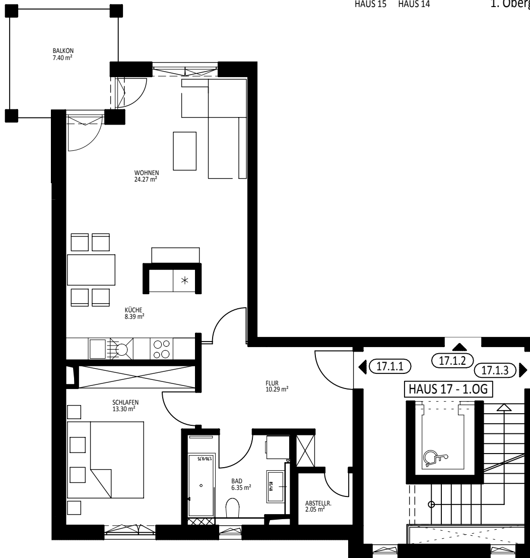
1. Obergeschoss
